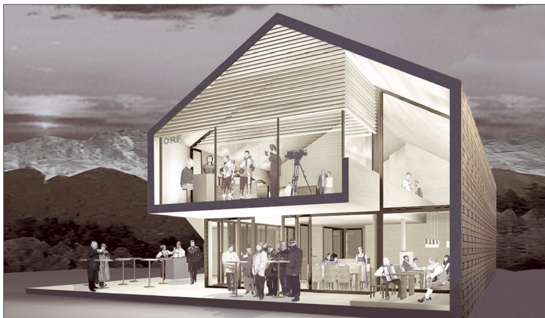
Das Österreichhaus, ein Projekt des Radstädter Architekturbüros „LP architektur“, repräsentiert unser Land bei Olympia in Turin. Der zerleg- und transportierbare Bau wird am 16. Februar um 13 Uhr von Architekt Thomas Lechner präsentiert und ist als Modell am Stand der Gemeindeentwicklung zu bestaunen.
